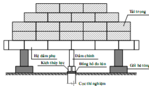
Hình A.1 - Gia tải bằng kích thủy lực, dùng dầm chất tải và đối trọng làm phản lực
