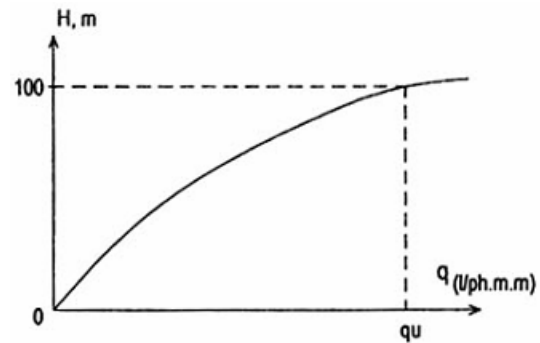
ĐỒ THỊ XÁC ĐỊNH TRỊ SỐ LUGEON CỦA ĐOẠN THÍ NGHIỆM H = F(Q)
