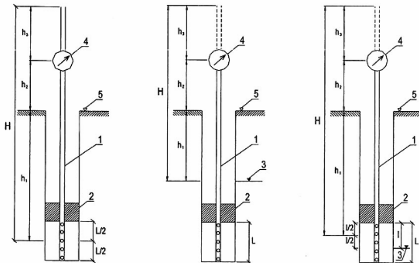
(a) đoạn thí nghiệm nằm trong đá không chứa nước
