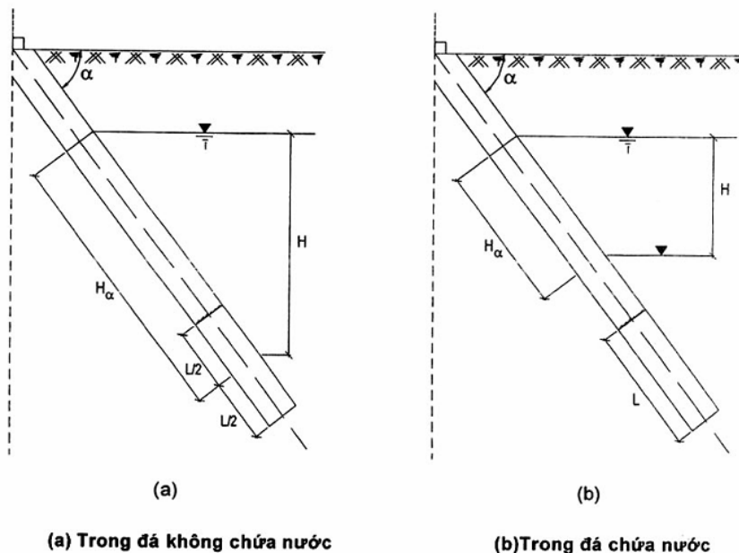
Hình 2 - Sơ đồ thí nghiệm ép nước trong lỗ khoan xiên
