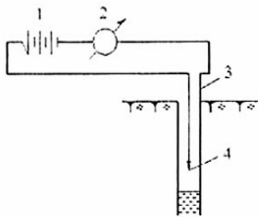
Hình B.3 - Sơ đồ dụng cụ mực nước bằng điện
